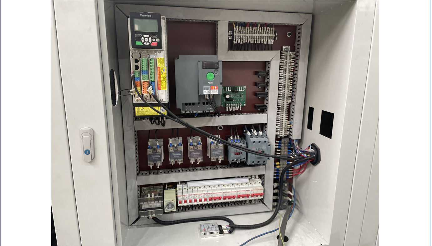
Kontrol Paneli
